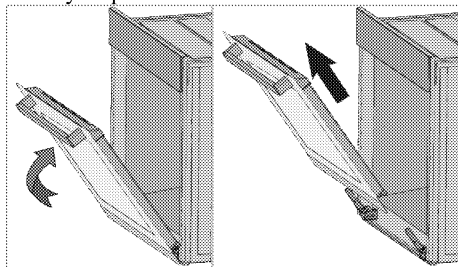
Шарнирный замок - открытое положение 3. Переведите дверцу духовки в полуоткрытое положение.
