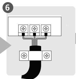
6 Ligar a cablagem (não aplicável em alguns locais nos Estados Unidos)
