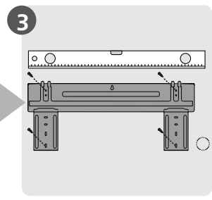
3 Fixar a placa de montagem
